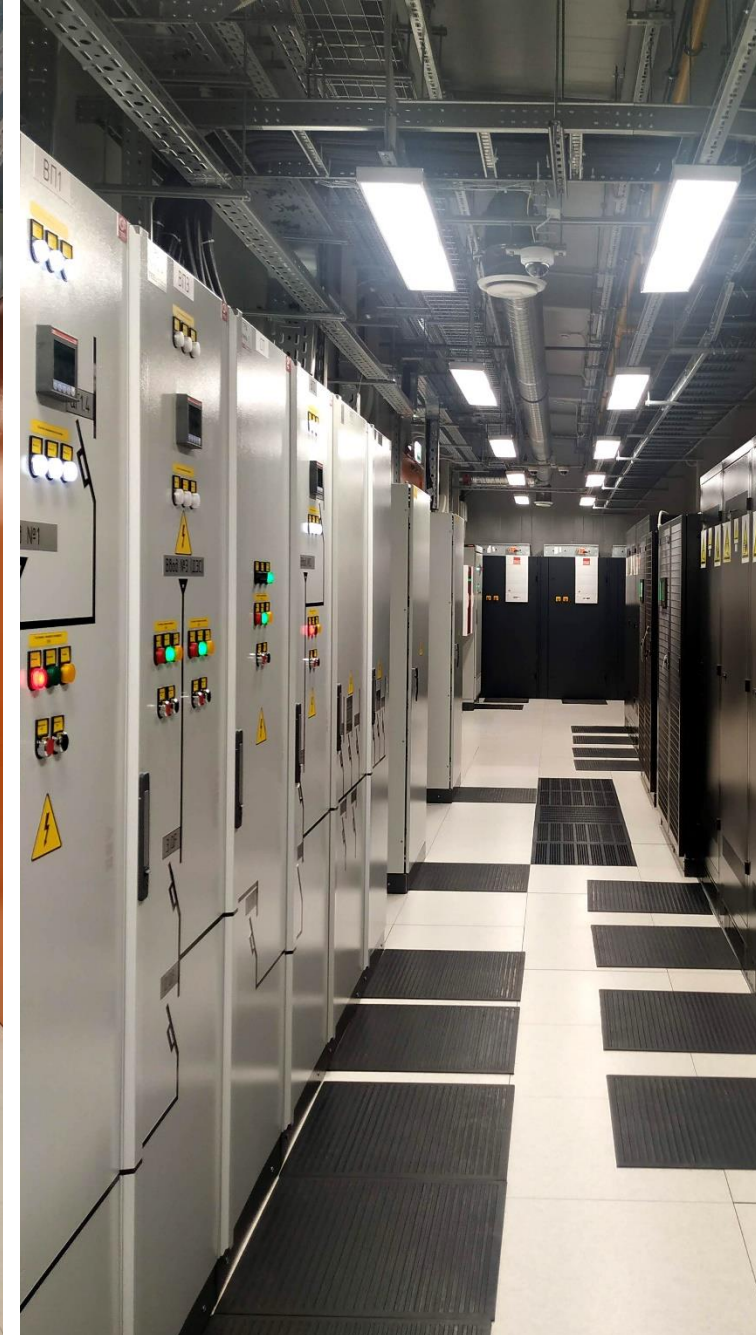
ЦОД «ПКК Миландр». Электрощитовая, ИБП, щитовое оборудование
